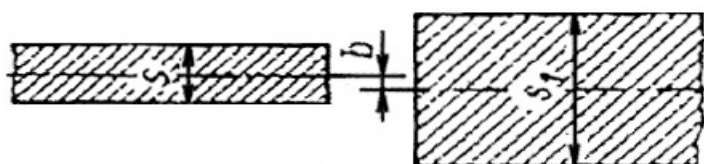
Рисунок 2. Смещение кромок листов
